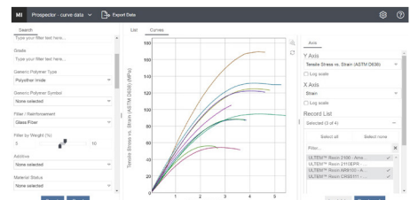
그림 3. 간단한 Granta MI 웹 앱에서 테스트 결과 비교
