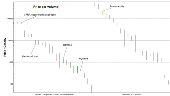
Gráfico: El carburo de boro y el CFRP presentan muy buen comportamiento, pero son caros. La madera es más barata.
