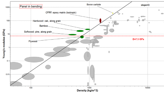
Gráfico: Materiales de igual o mejor (por encima de la recta de visualización) comportamiento que el contrachapado.
